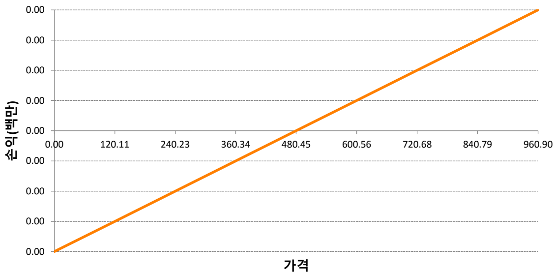
KR4101WC0003-2025-12 코스피200지수선물
